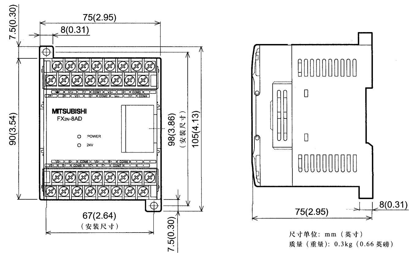
图 2.1: 外部尺寸
