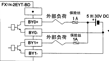
源型
