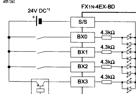
源型
