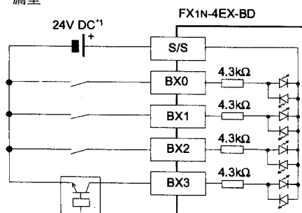
漏型
