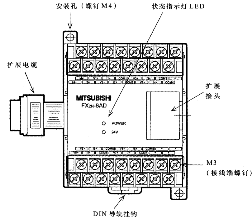
图 3.1: 部件名字
