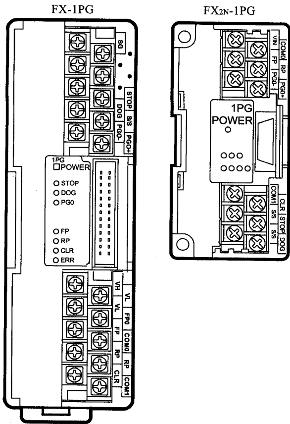
<LED 分配>
