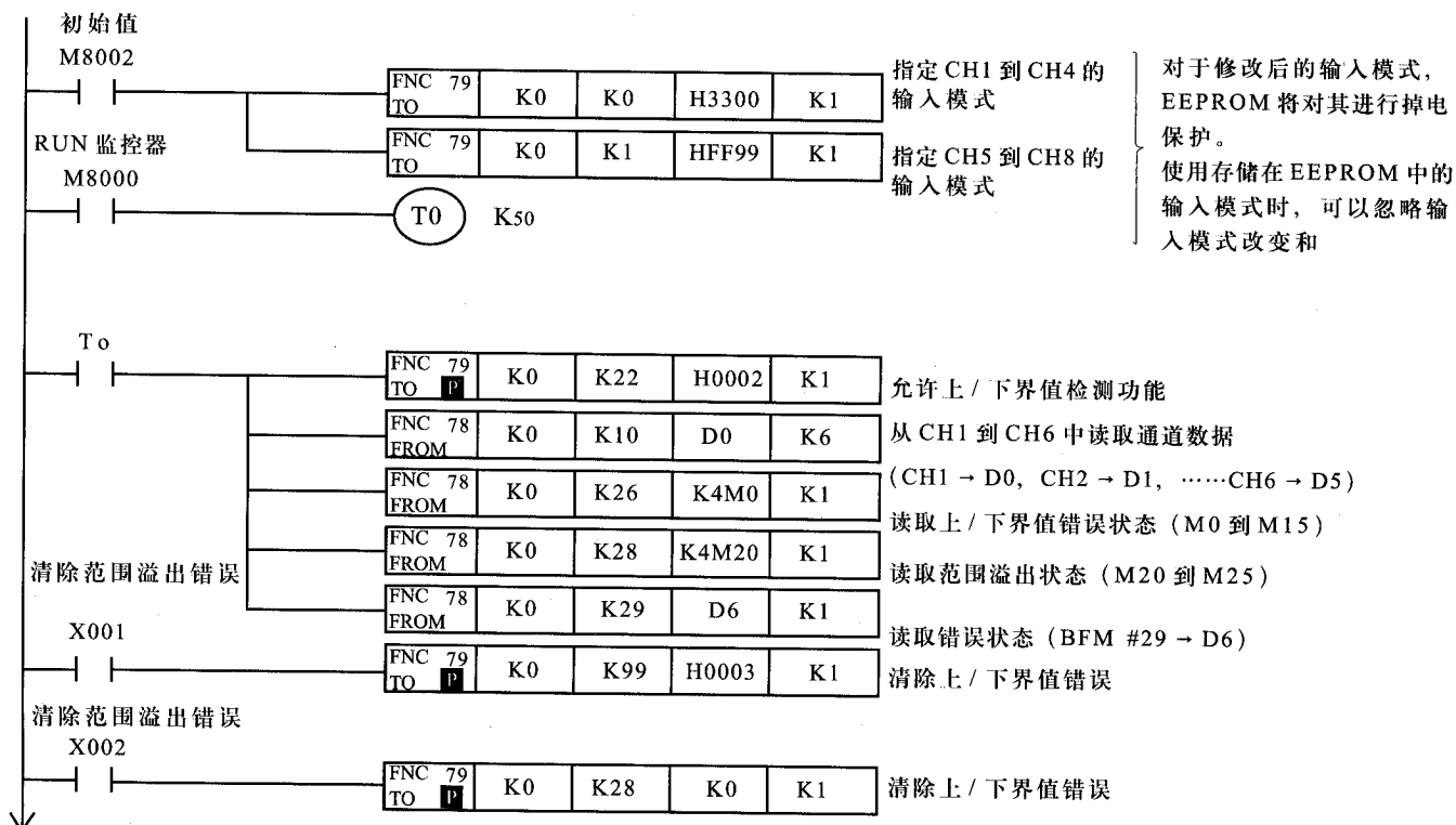
图 10.1: 实例程序
