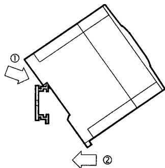
FX 2N 2LC 接到 DIN 导轨上时
