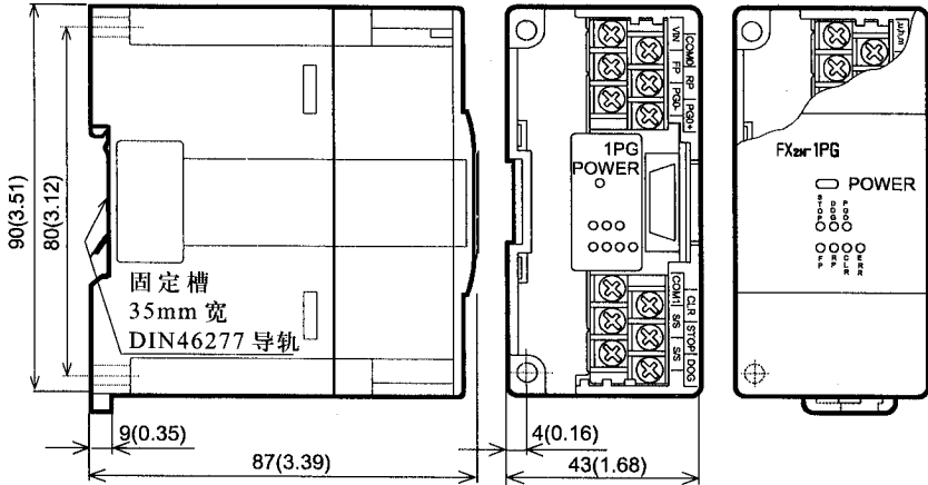
FX 2N -1PG
