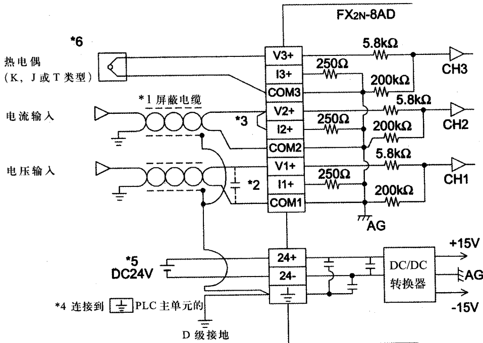
图 6.2: 配线
