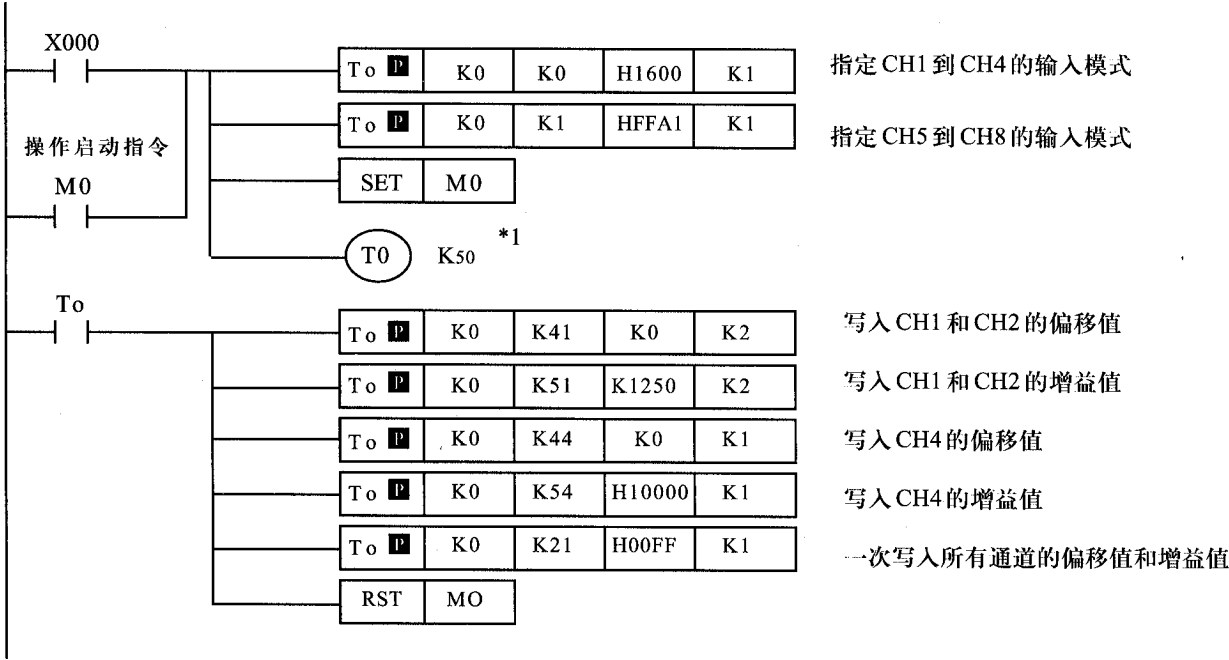
图9.2：实例程序
